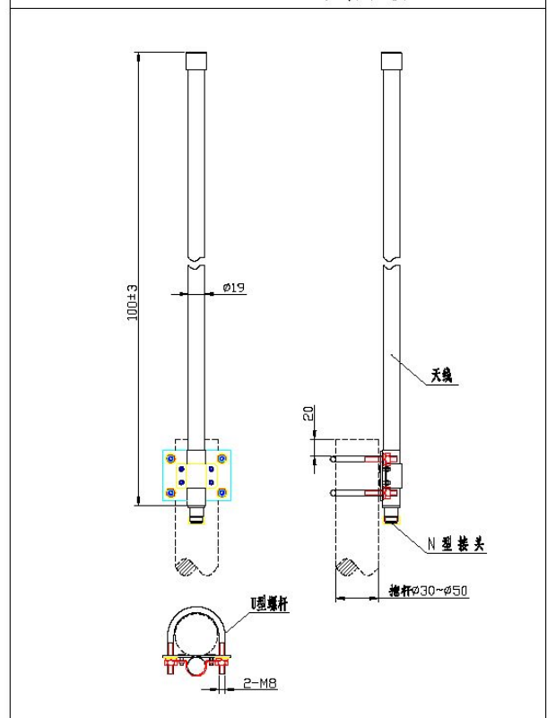
TQJ - 1400AT8 安装示意图
