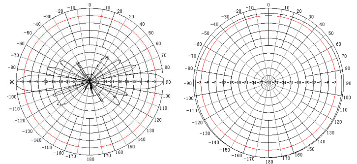
E 面方向图
