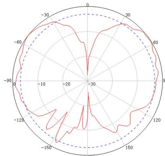
典型 E 面方向图
