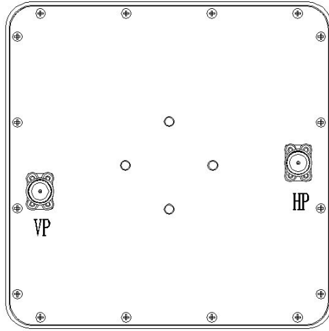
安装示意图
