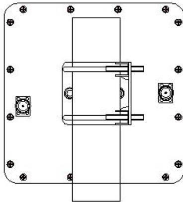
安装示意图
