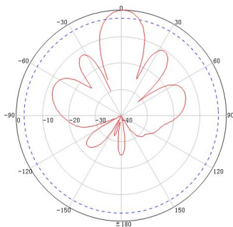
5150-58500MHZ 水平面
