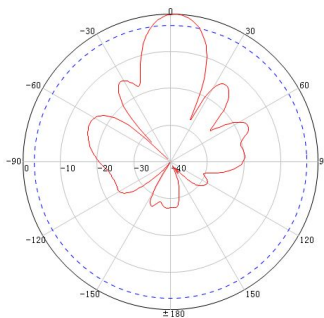
5150-5850MHZ 垂直面
