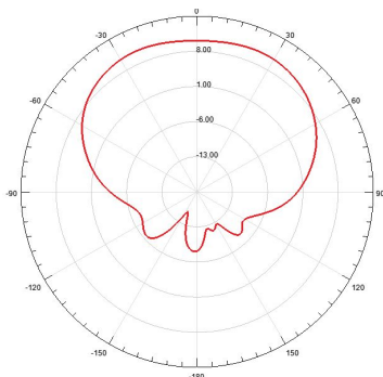
水平面参考方向图
