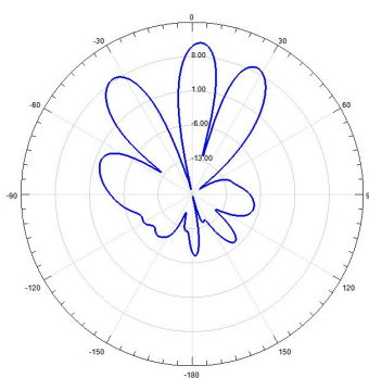
垂直面参考方向图
