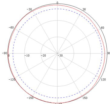
700~840MHz 典型 H 面方向图:
