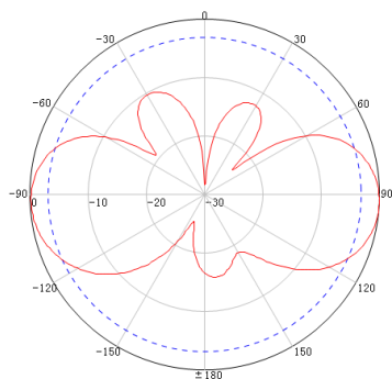
700~840MHz 典型 E 面方向图:
