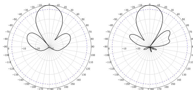
2.4G 参考方向图 H 面/E 面
