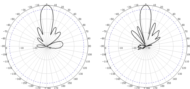
5G 参考方向图 H 面/E 面
