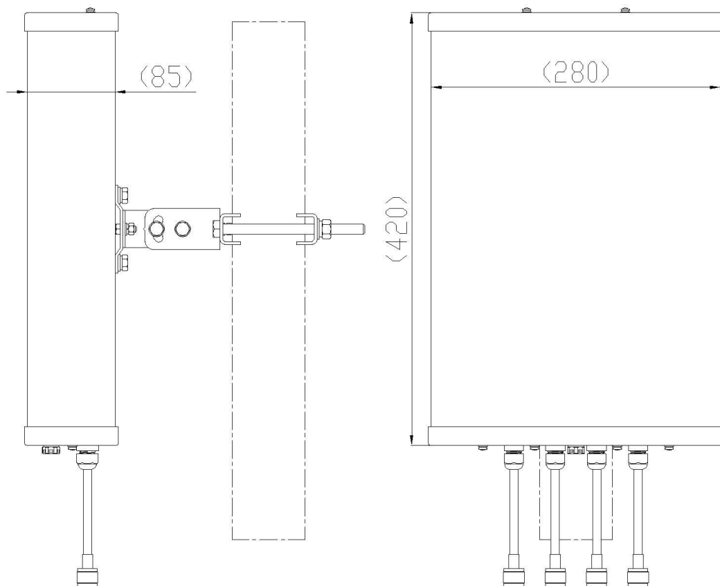
天线尺寸/安装示意图
