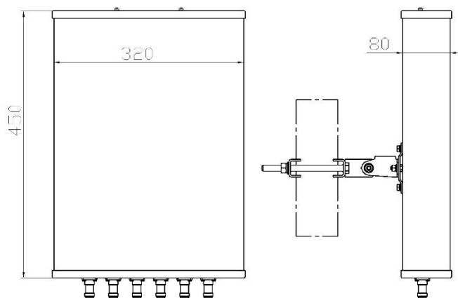
安装示意图
