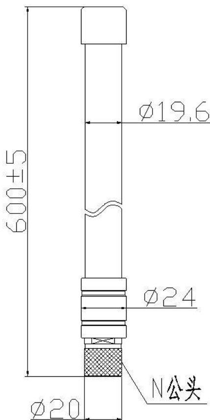
外形尺寸图
