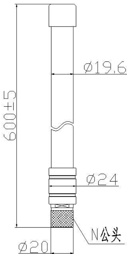
外形尺寸图
