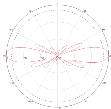
典型 E 面方向图
