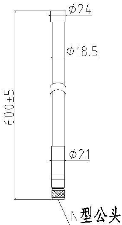
产品外形尺寸图
